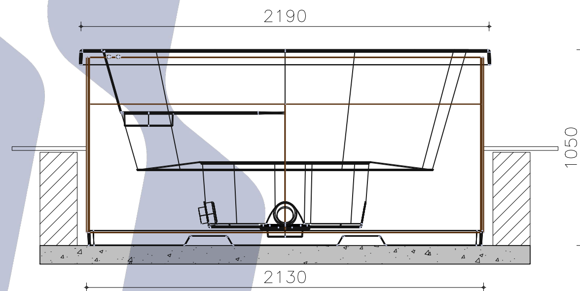
Aanzicht A-A
