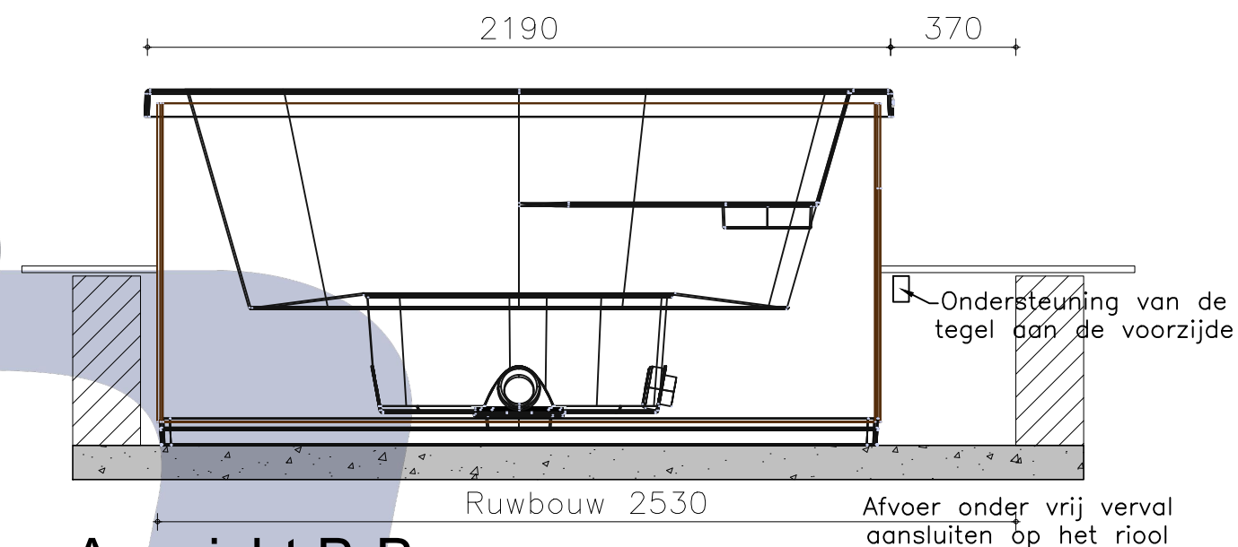
Aanzicht B-B
