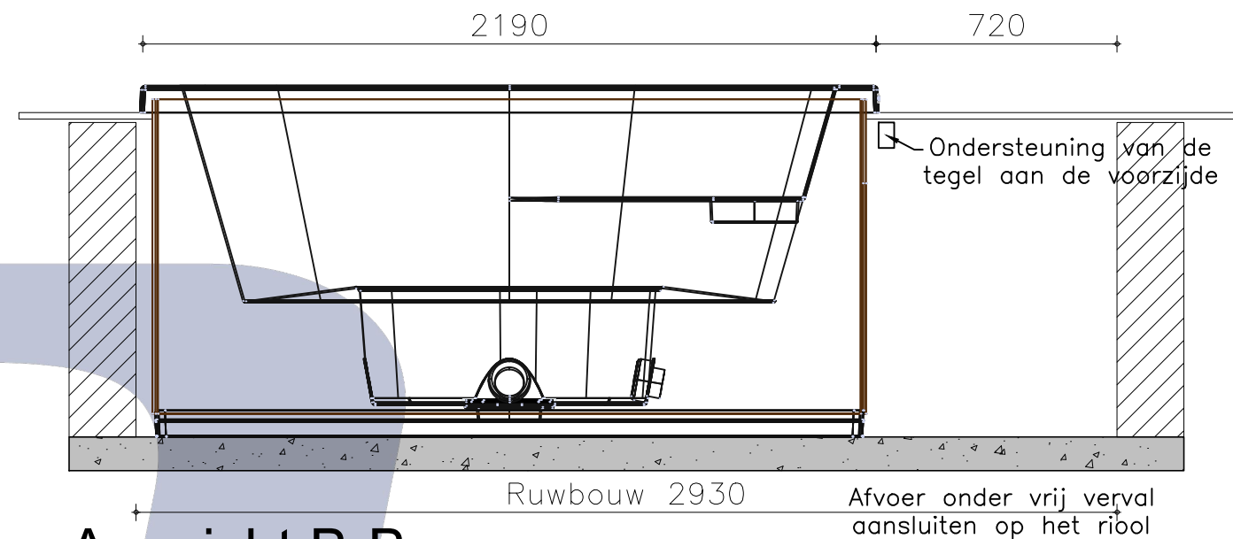
Aanzicht B-B
