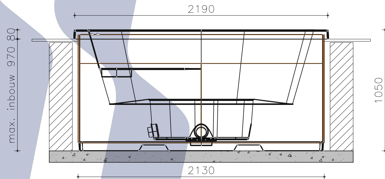
Aanzicht A-A
